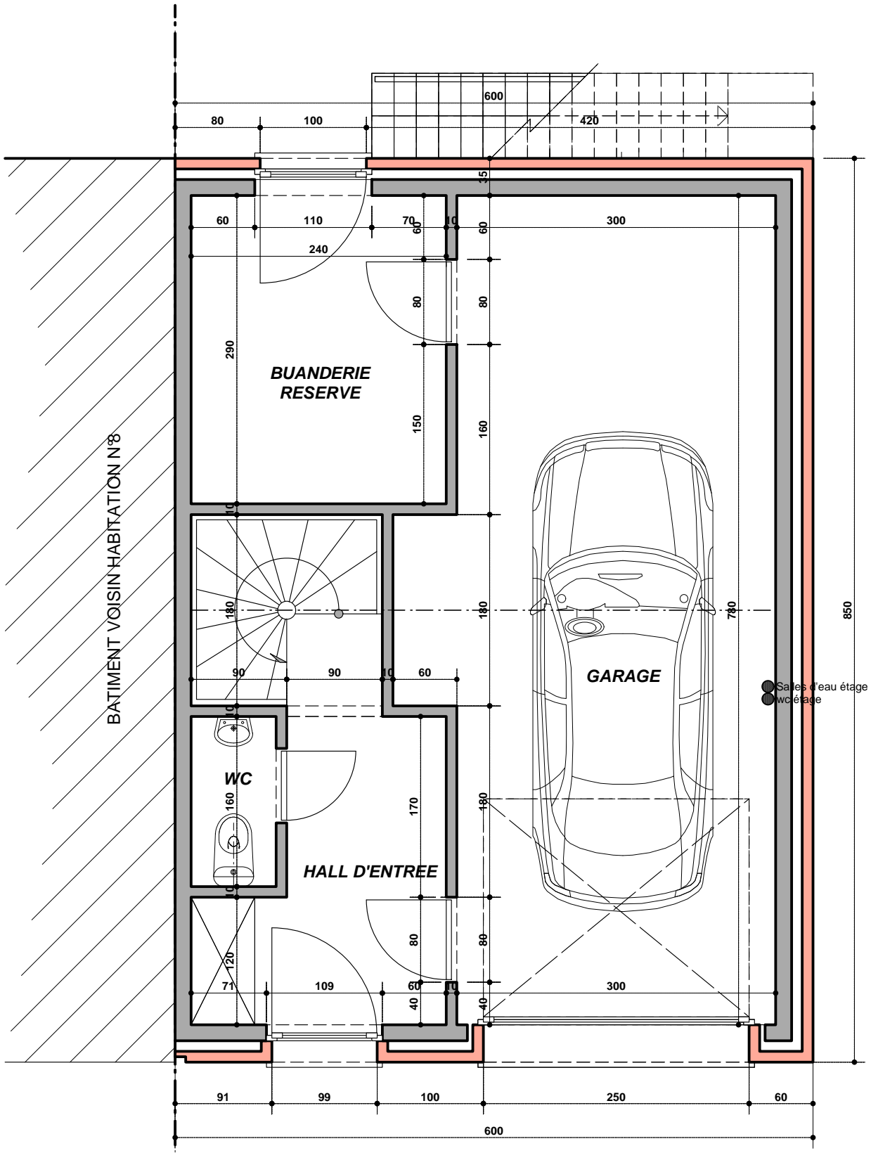
REZ - DE - CHAUSSEE ECHELLE 1/50
